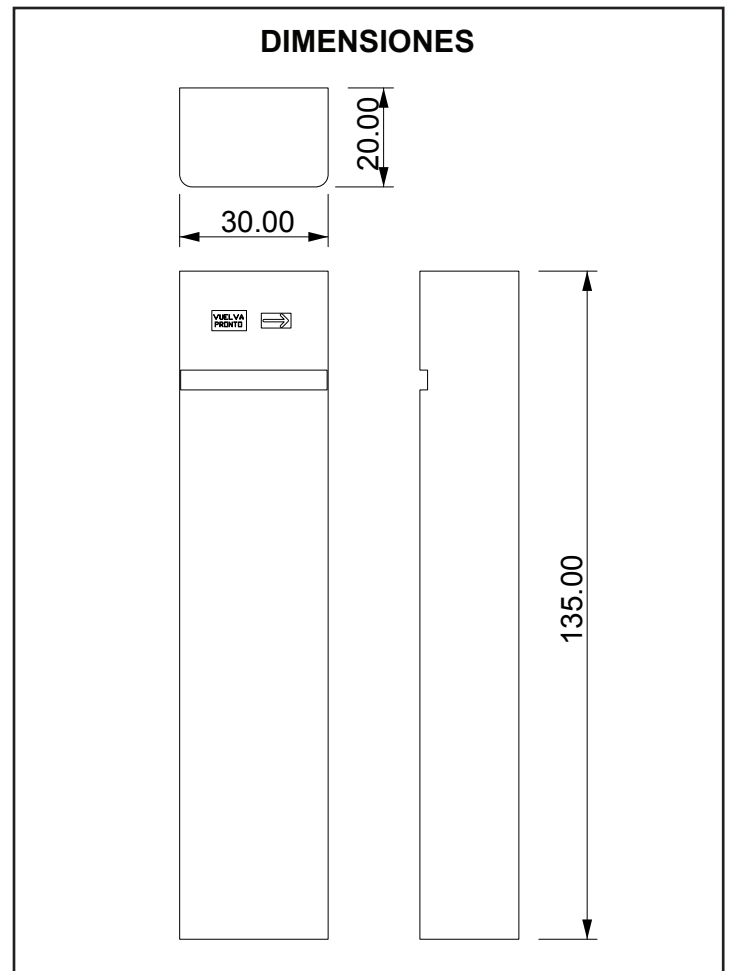
VISTA GENERALES DEL VALIDADOR DE BOLETOS. ACOTADO EN CM
